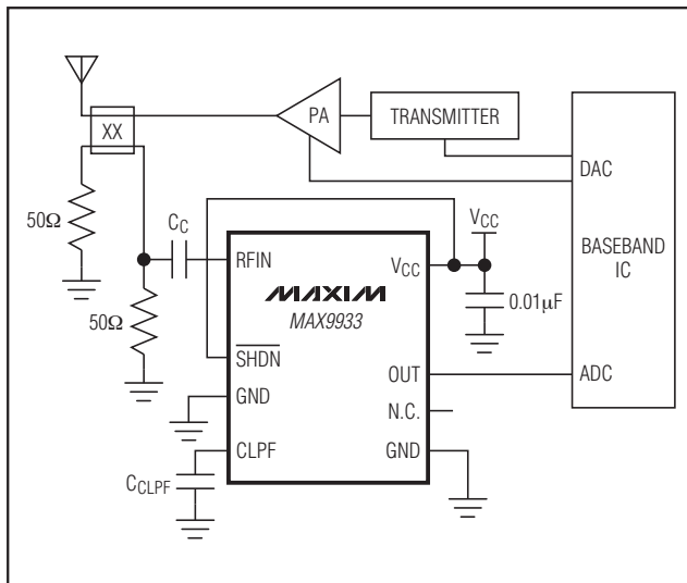
図2. MAX9933の標準動作回路
