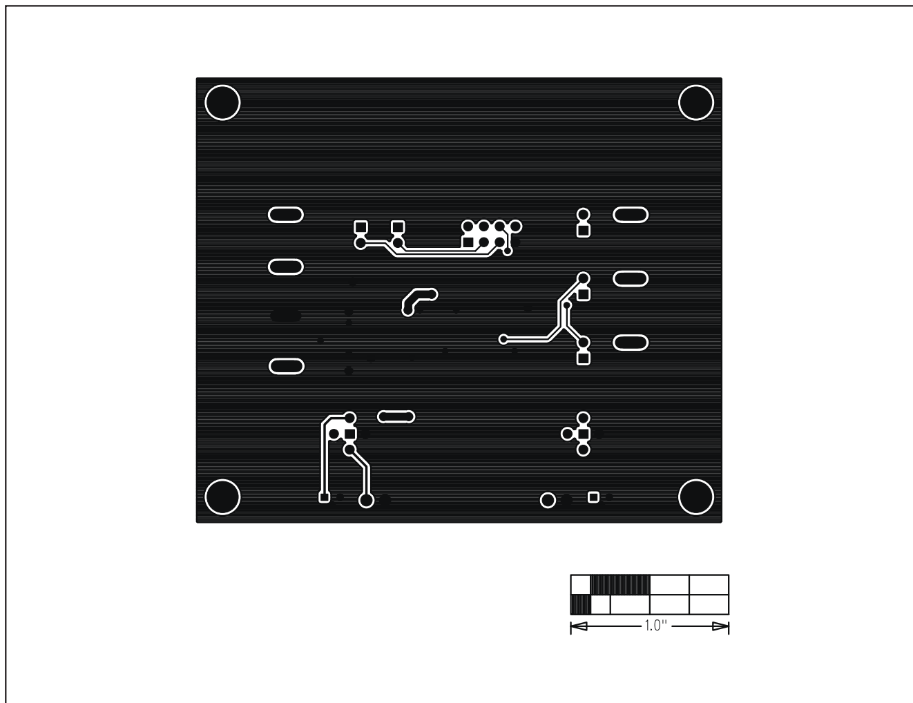
図4. MAX9921のEVキットのPCBレイアウト—半田側
