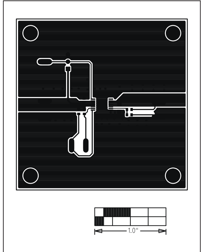
図3. MAX8526のEVキットのPCBレイアウト—部品面
