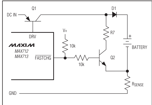
図7. NiMHバッテリー用のトリクル充電電流の抑制(リニアモード)
