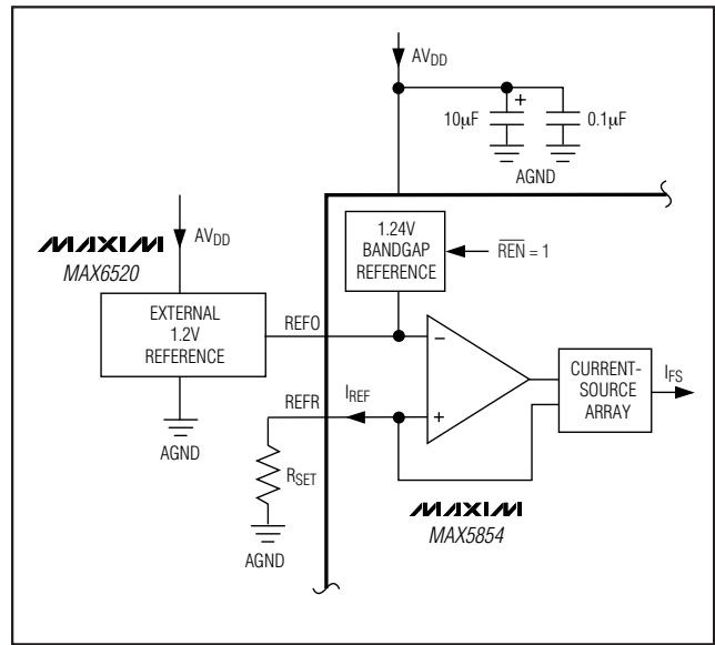
図4. 外部リファレンス付MAX5854
