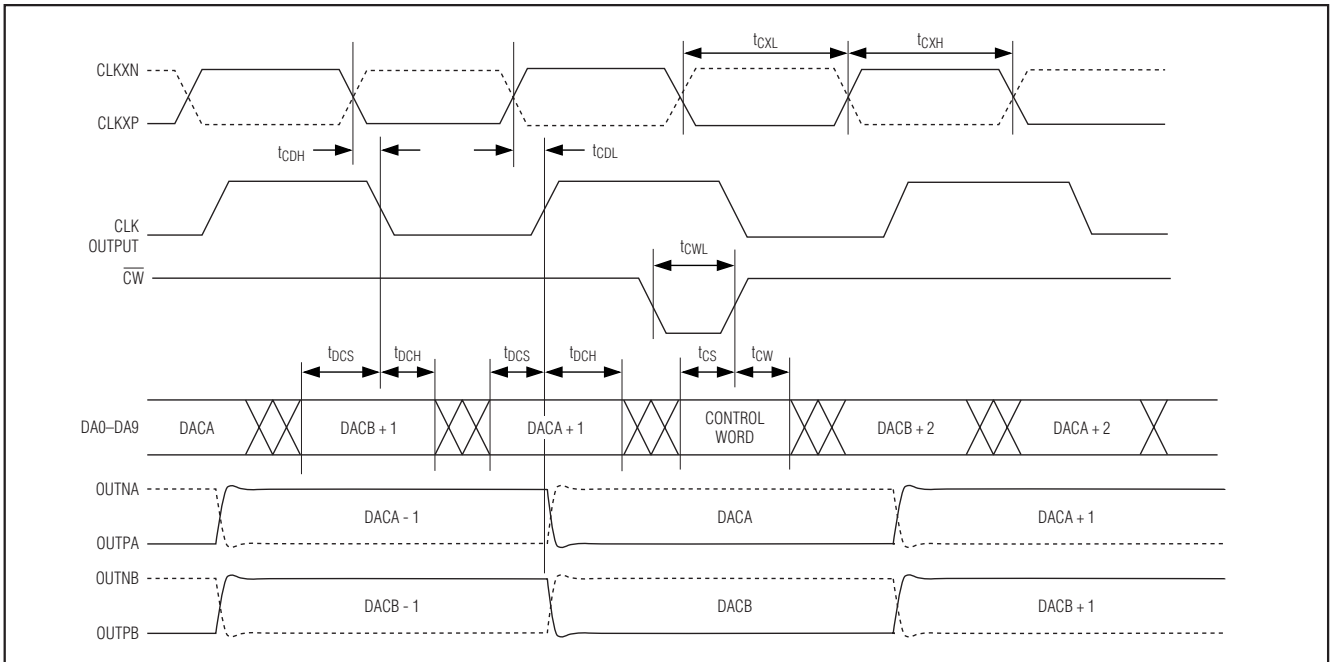
図6. インタリーブデータモードのタイミング図 (IDE = 1)
