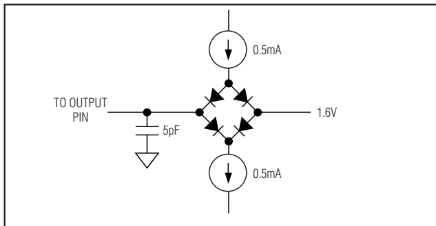
図1. CLK出力用の負荷試験回路
