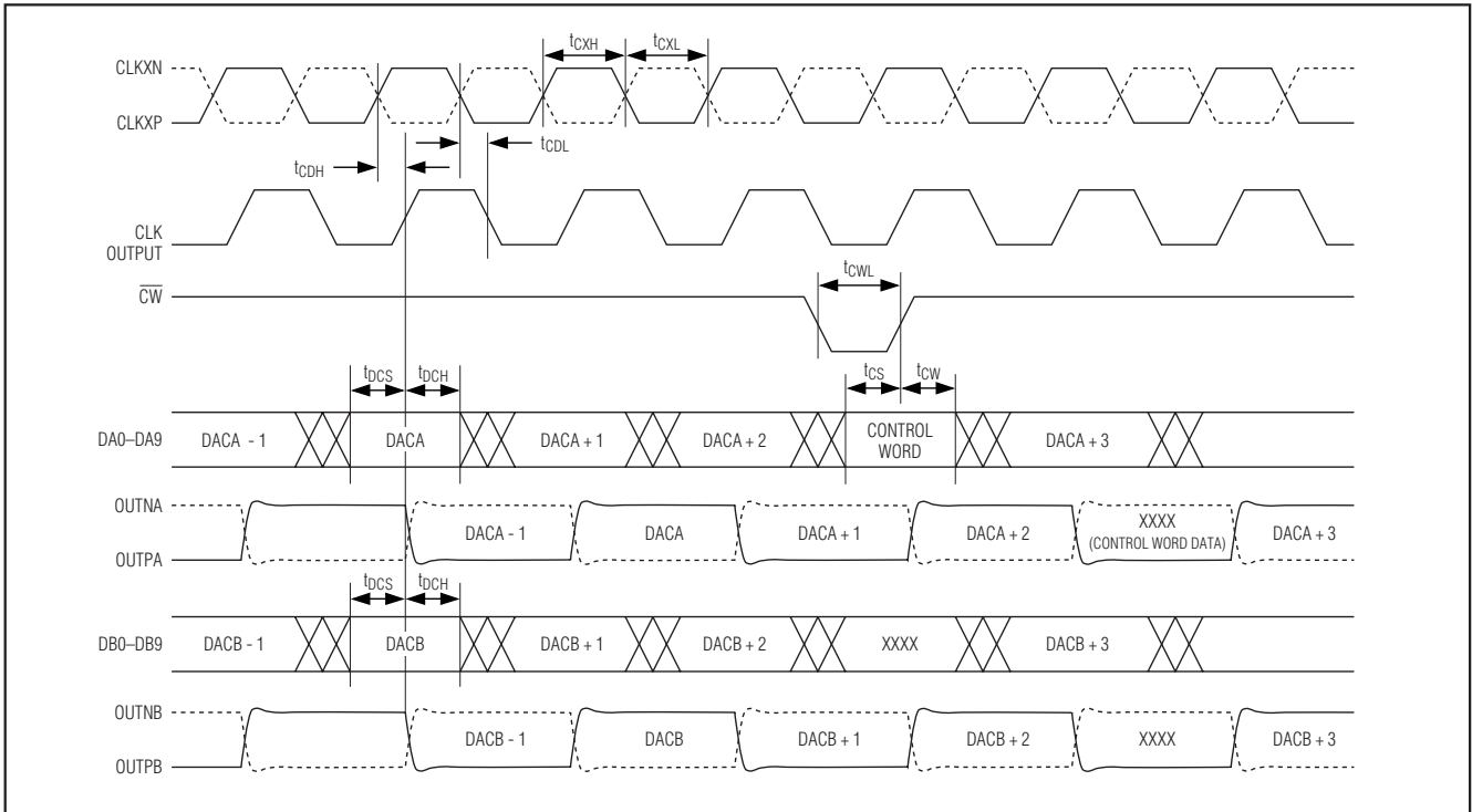
図5. 非インタリーブデータモードのタイミング図 (IDE = 0)
