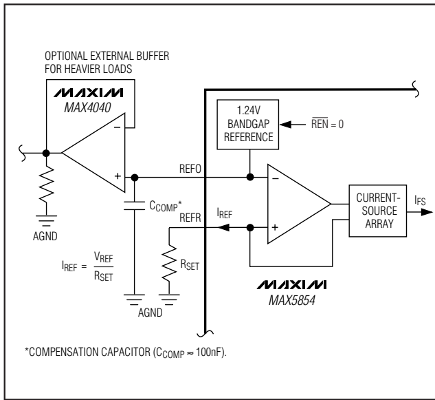
図3. 1.24V内部リファレンス及び制御アンプによる I_{FS} の設定
