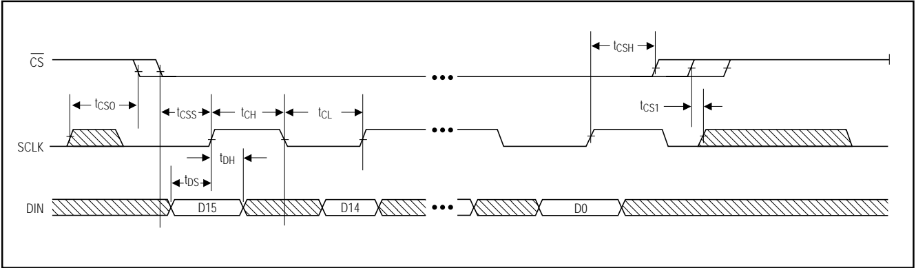
図3. 3線シリアルインタフェースのタイミング図
