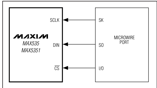
図2. Microwire用の接続
