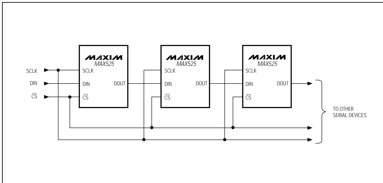
図7. MAX525のデジーチェーン接続
