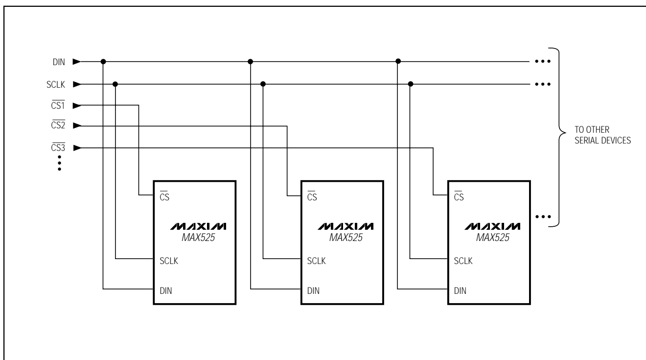
図8. 複数のMAX525がコモンDINラインを共有
