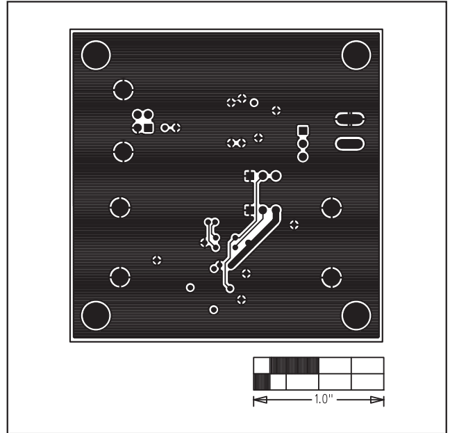
図7. MAX4983EのEVキットのPCBレイアウト—半田面
