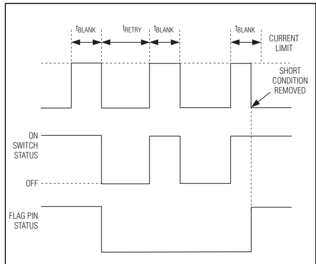
図2. MAX4796/MAX4798の自動再試行障害ブランキング図
