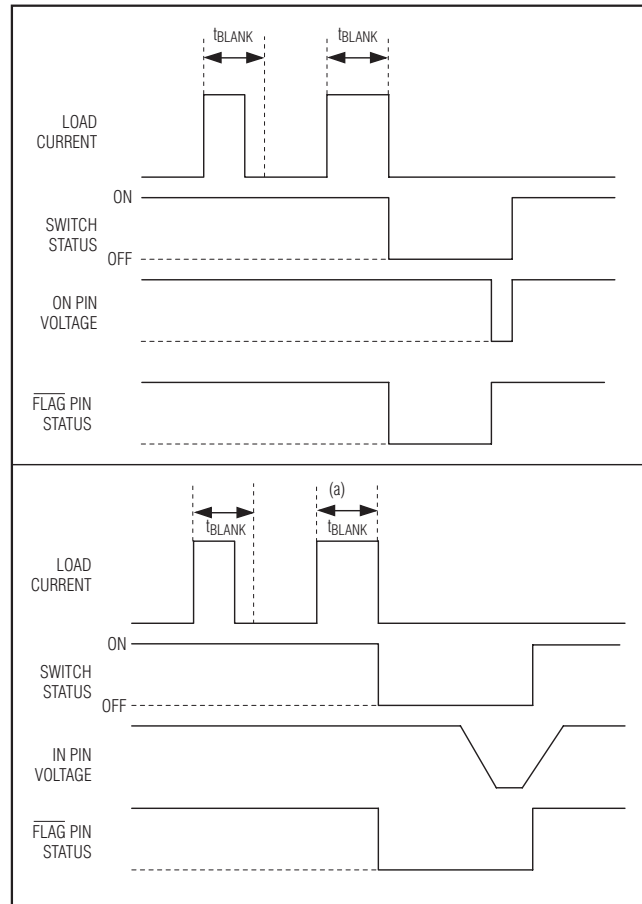
図3. MAX4795/MAX4797のラッチオフ障害ブランキング
