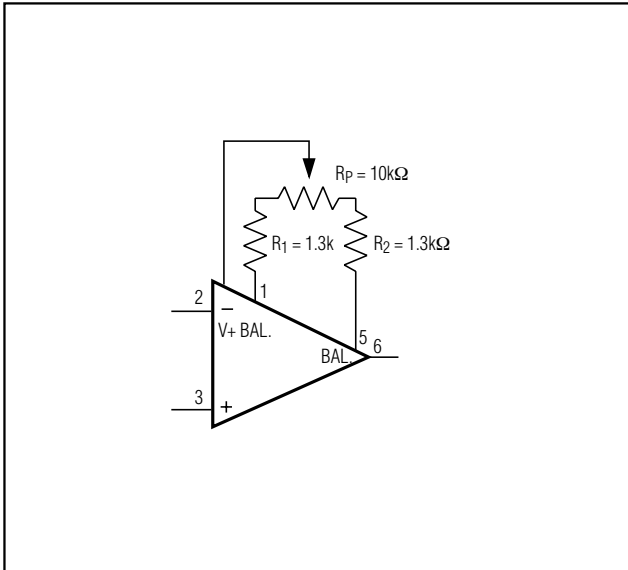
図2. MAX408の V_{OS} のヌル調整方法
