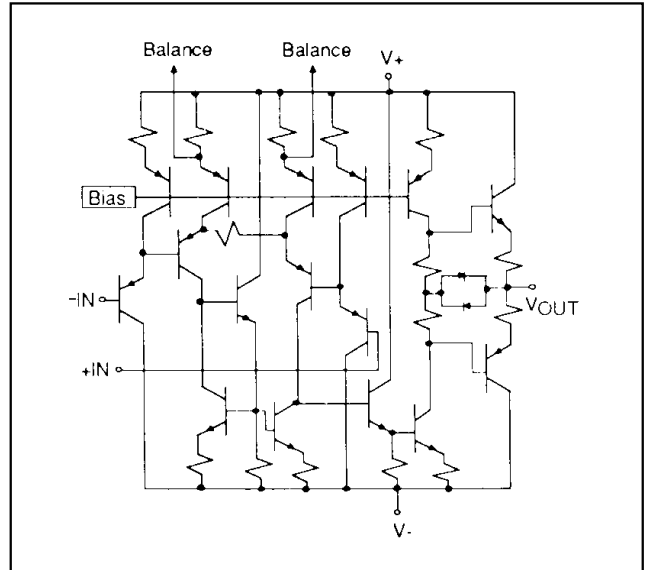
簡略化回路図。MAX428/448の場合はバランスピンを外して下さい。
