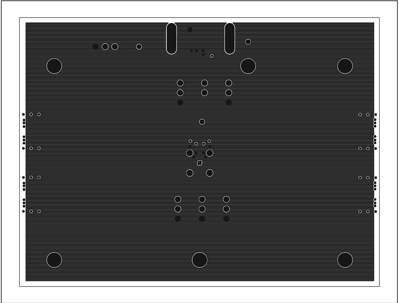
図6. MAX3984のEVキットのPCBレイアウト—電源プレーン、第3層
