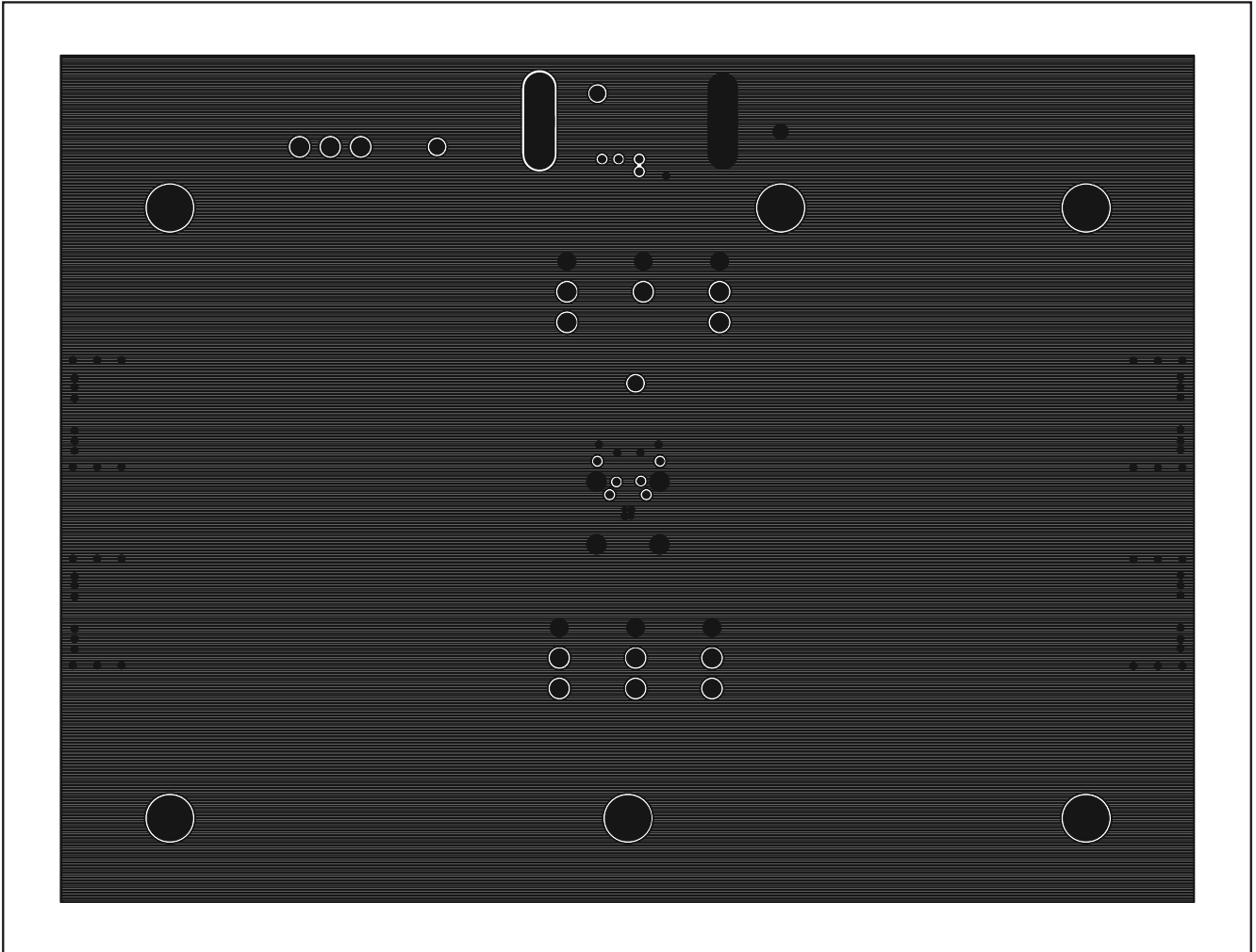
図5. MAX3984のEVキットのPCBレイアウト—グランドプレーン、第2層
