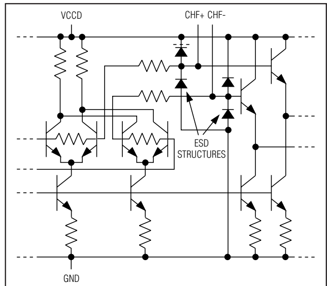
図6. CHFパッド
