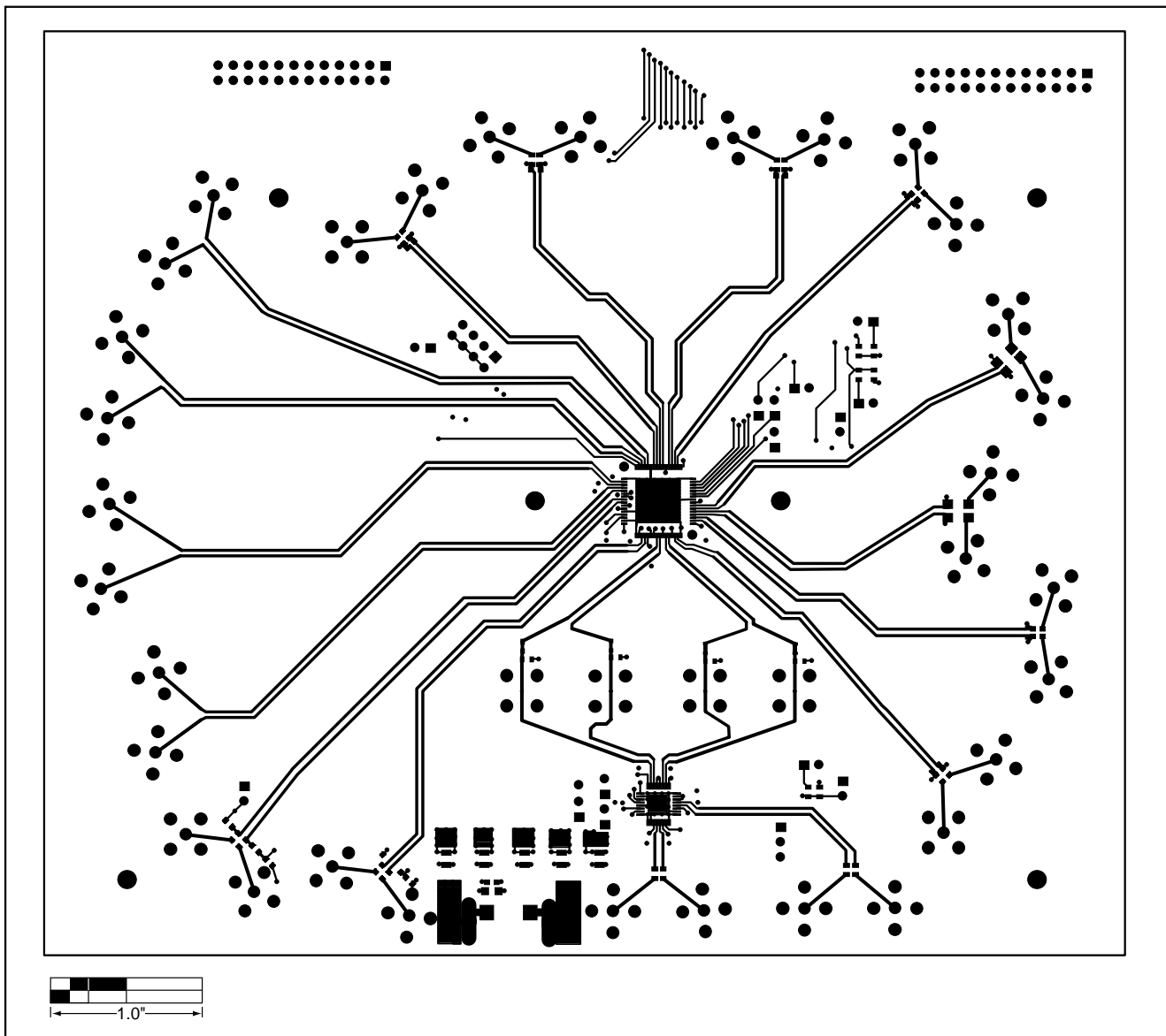
図4. MAX3831/MAX3832EVキットのプリント基板レイアウト(部品面側)
