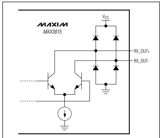
図5. 簡略化した出力回路図
