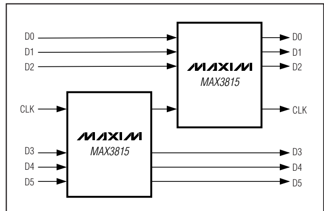
図2. MAX3815をDual Linkアプリケーションに使用する場合の接続図
