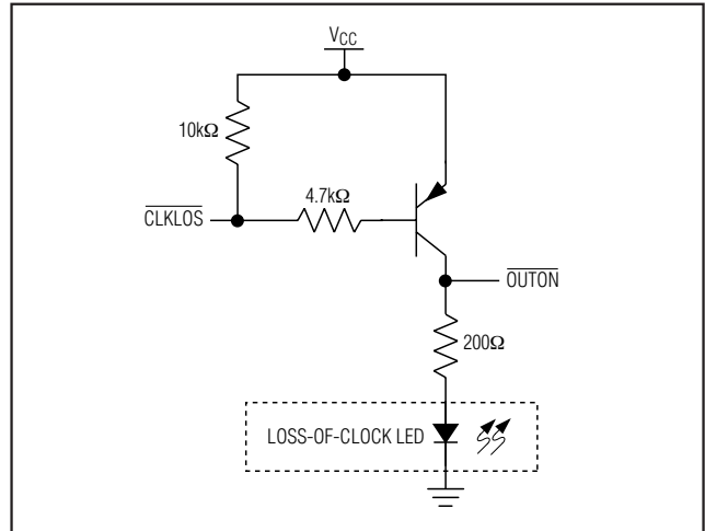
図3. スケルチ回路
