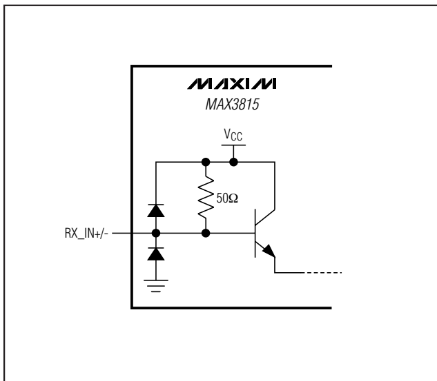
図4. 簡略化した入力回路図
