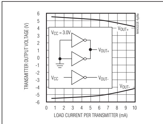
図6a. MAX3241Eのトランスミッタの出力電圧とトランスミッタ1つ当りの負荷電流の関係
