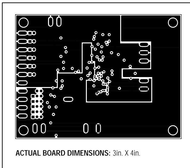
図5. MAX1802EVキットのプリント基板レイアウト -- V CC 層3
