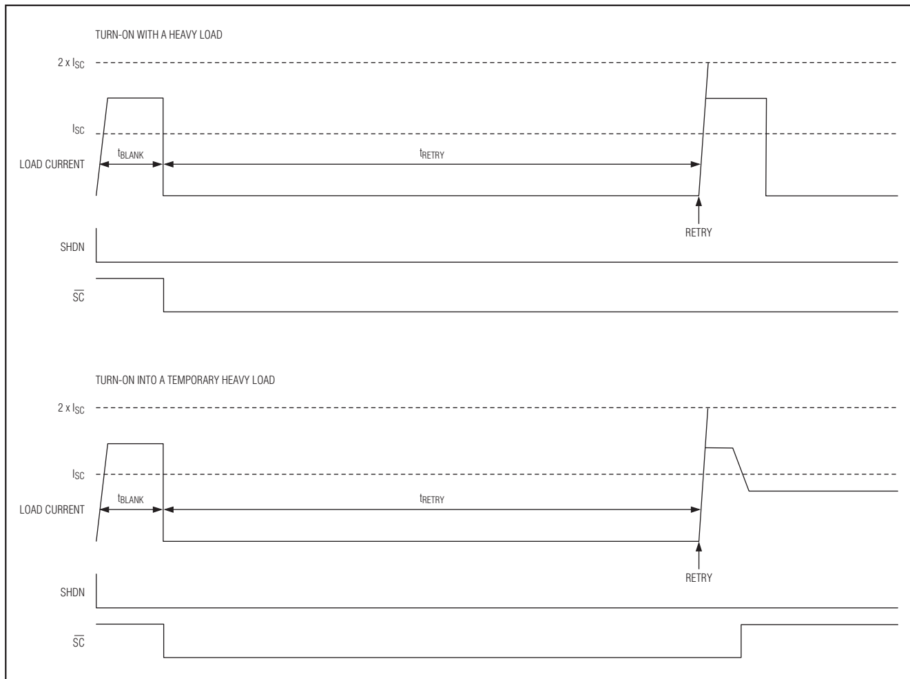
図2. 過電流のタイミング図
