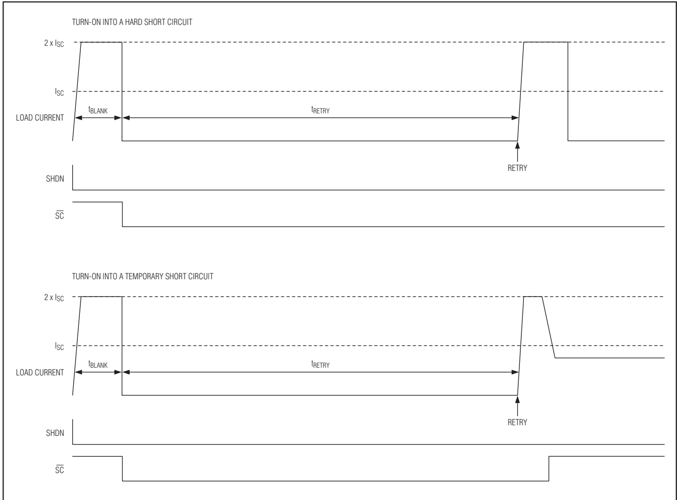
図1. 短絡のタイミング図
