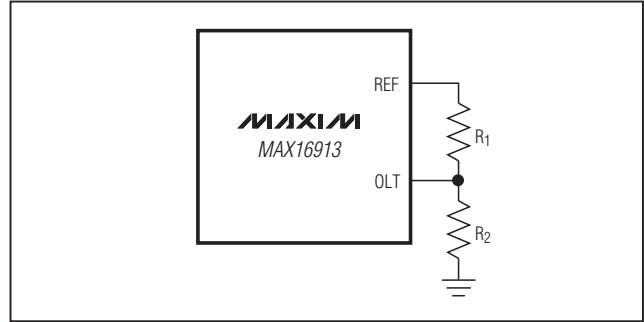
図3. オープン負荷スレッショルドの選択
