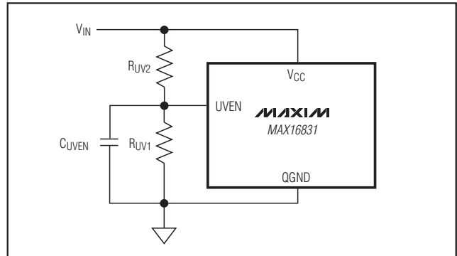
図1. UVLOスレッショルドの設定
