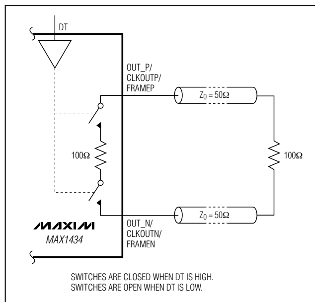
図8. 2重終端
