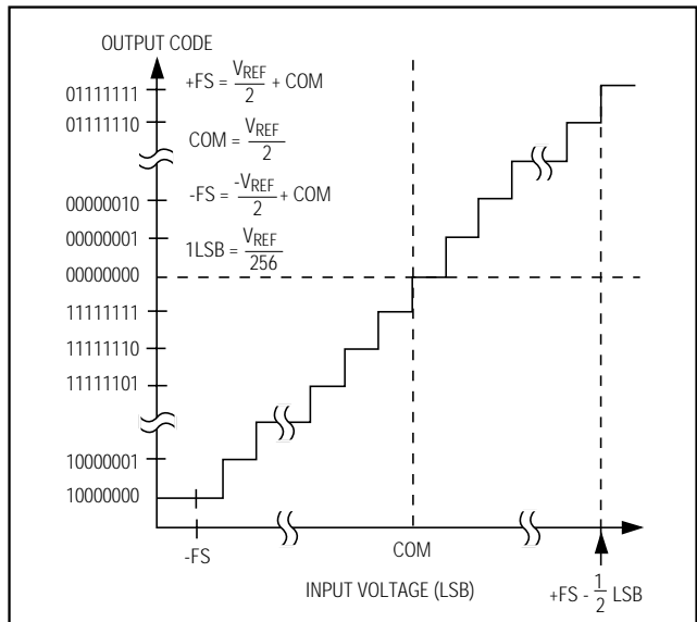
図12b. バイポーラ伝達関数
