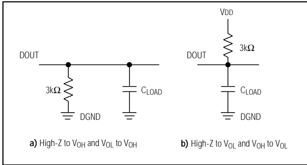
図1. イネーブル時の負荷回路
