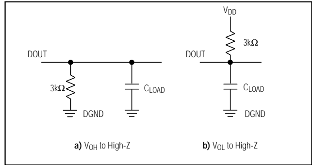
図2. ディセーブル時の負荷回路
