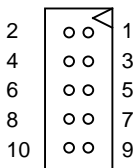
图7. IDC 连接器
