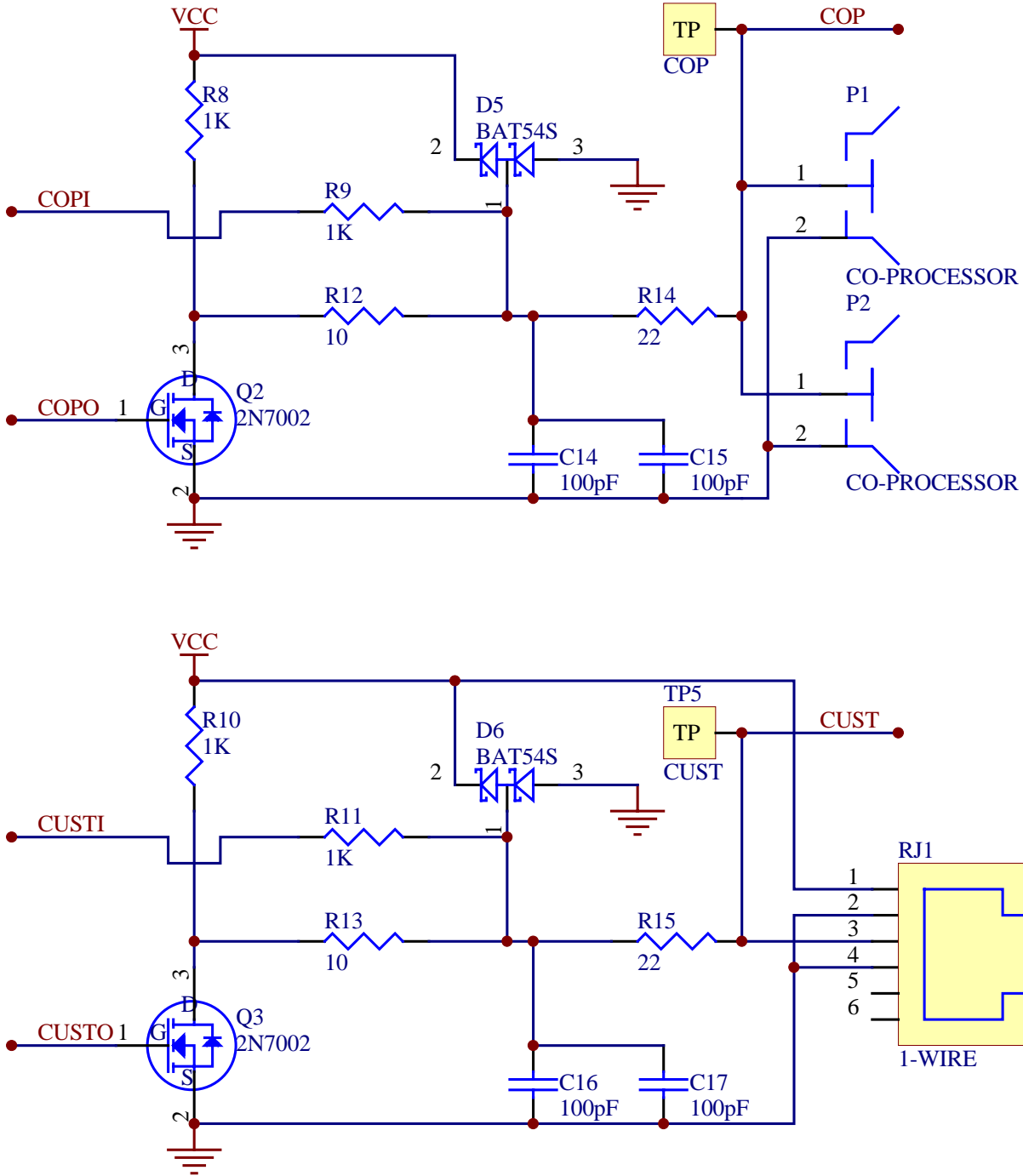
图13. 协处理器和 1-Wire 客户端电路
